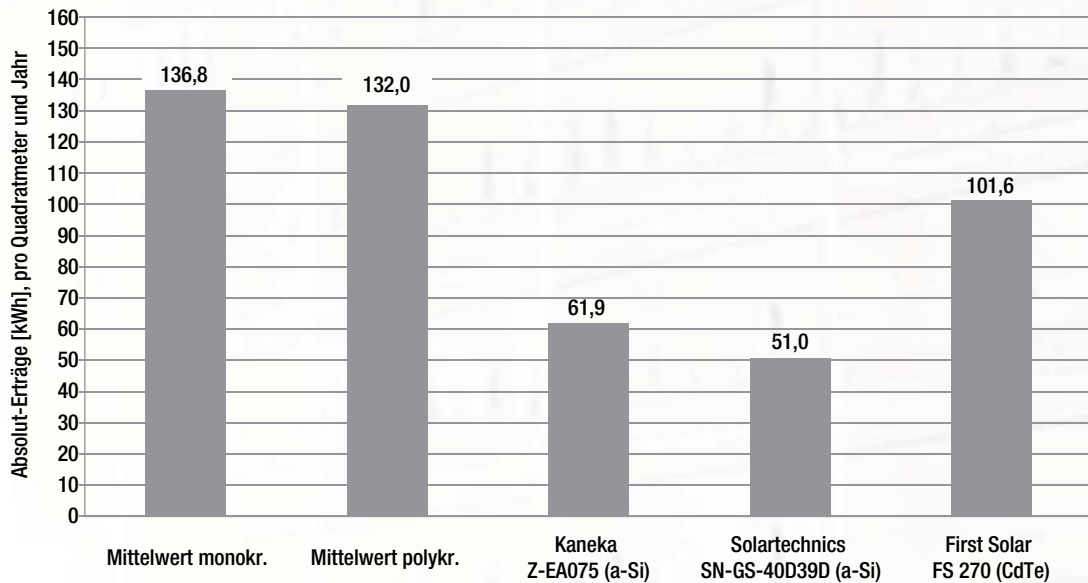
Abb. 7: Absolut-Erträge der verschiedenen Zellenarten (kWh), pro m 2 , 01.10.2008 bis 30.09.2009
