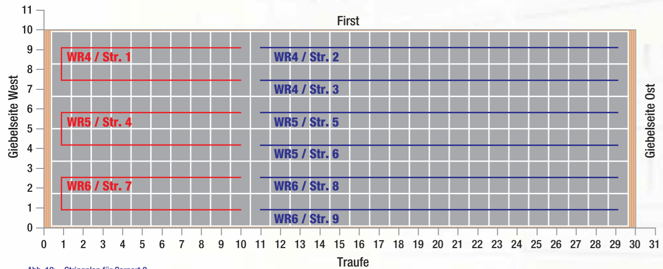
Abb. 12: Stringplan für Carport 2
